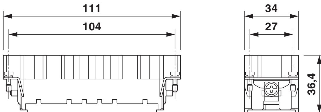
Rysunek wymiarowy
