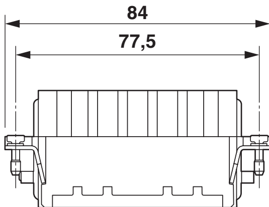
Rysunek wymiarowy
