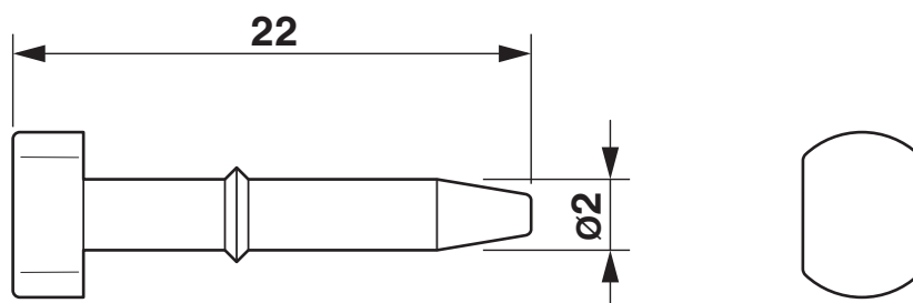
Rysunek wymiarowy
