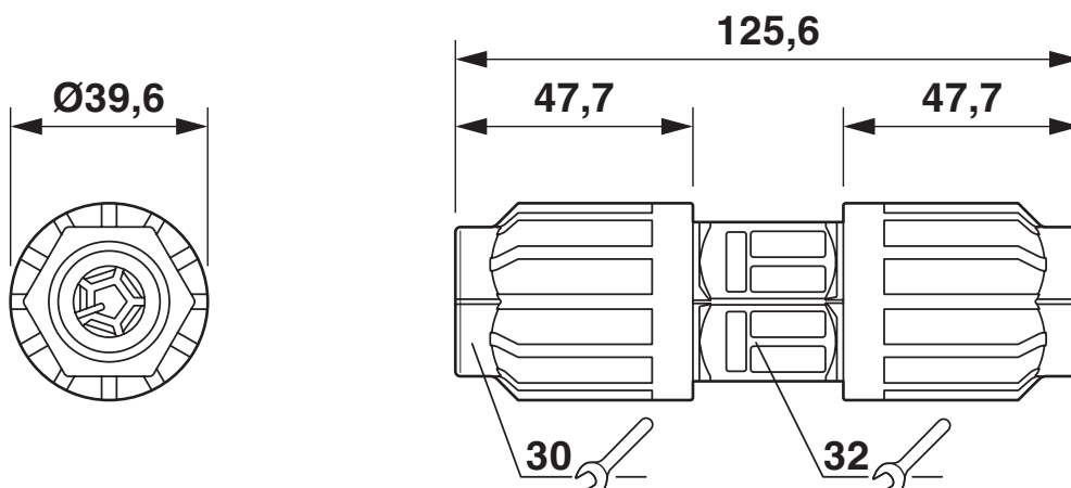
Rysunek wymiarowy QPD C 5x6,0
