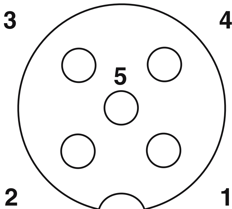
Rysunek schematyczny
