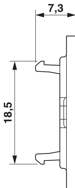
Rysunek wymiarowy
