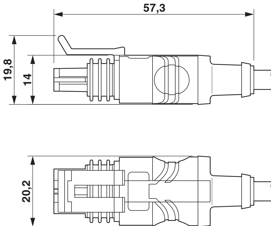
Rysunek wymiarowy
