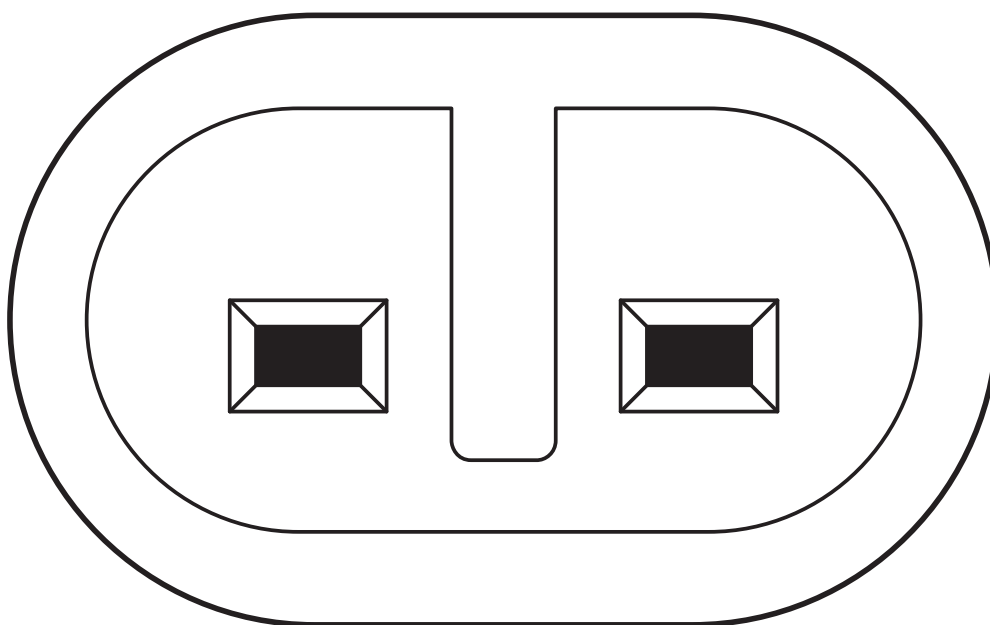
Układ styków 2-pinowego gniazda Super Seal
