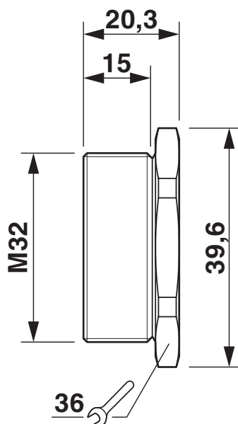
Rysunek wymiarowy
