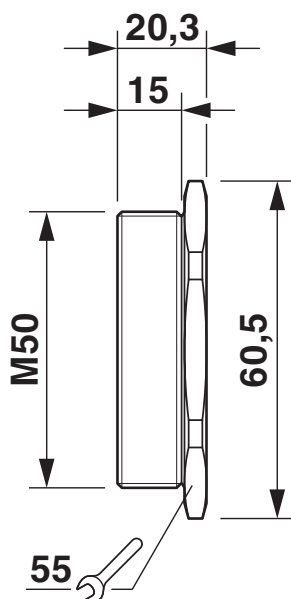
Rysunek wymiarowy
