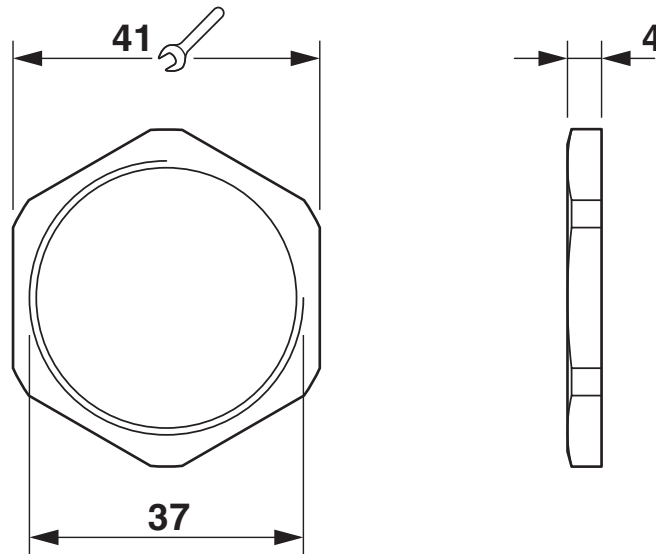
Rysunek wymiarowy
