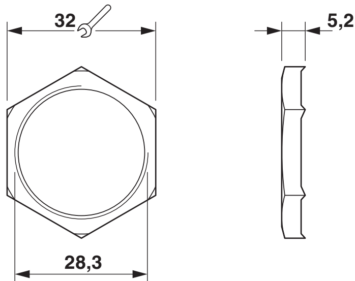
Rysunek wymiarowy
