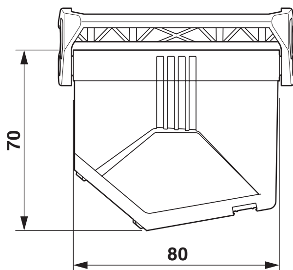
Rysunek wymiarowy
