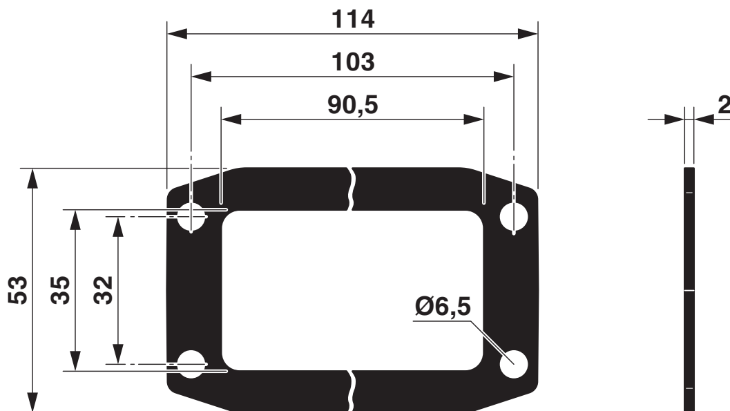
Rysunek wymiarowy
