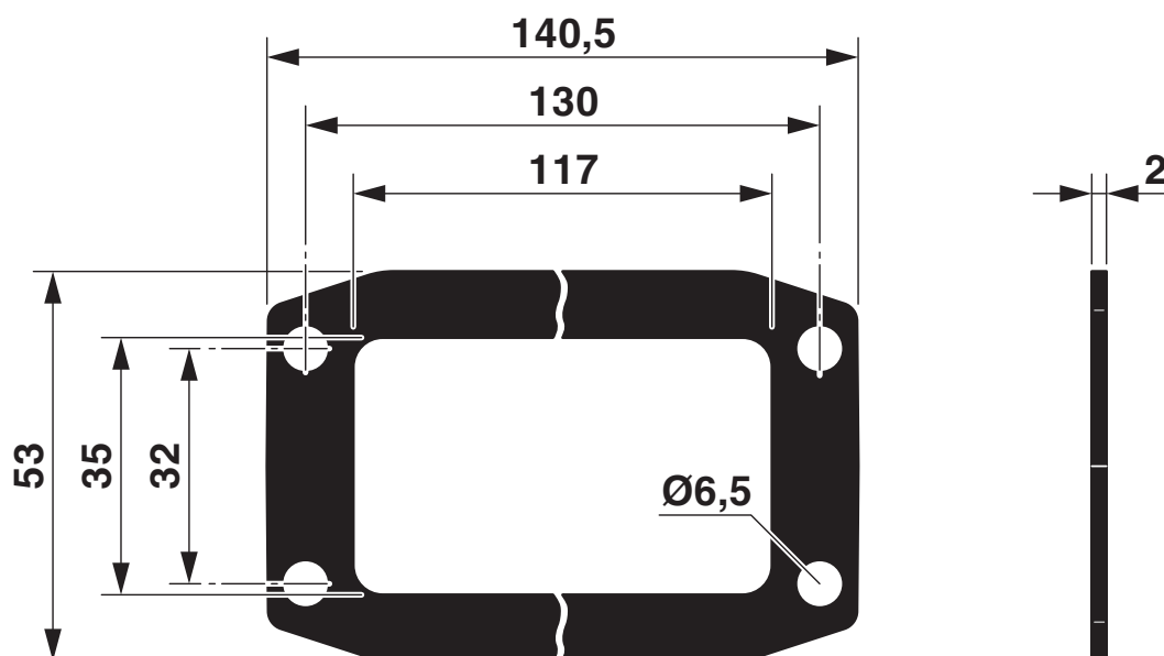
Rysunek wymiarowy
