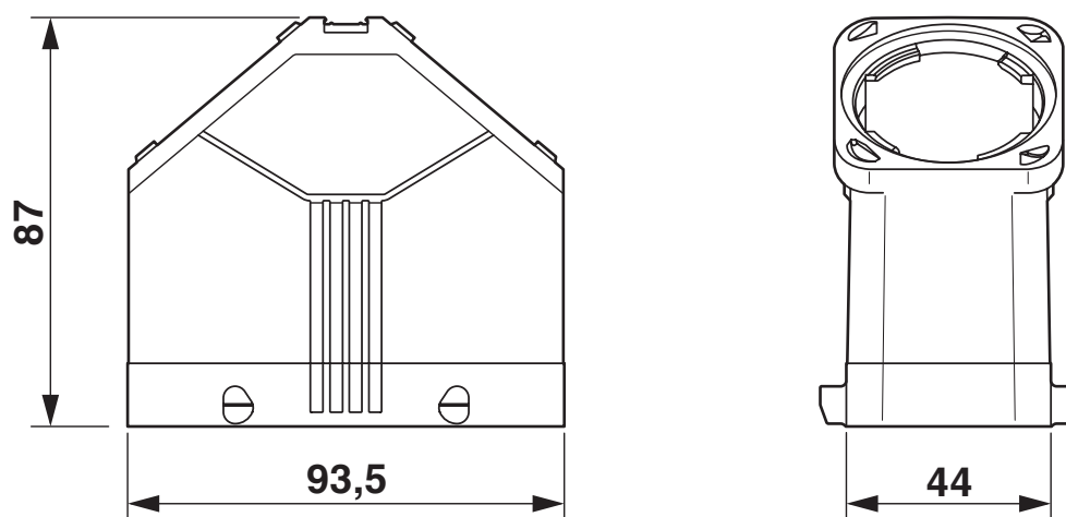
Rysunek wymiarowy
