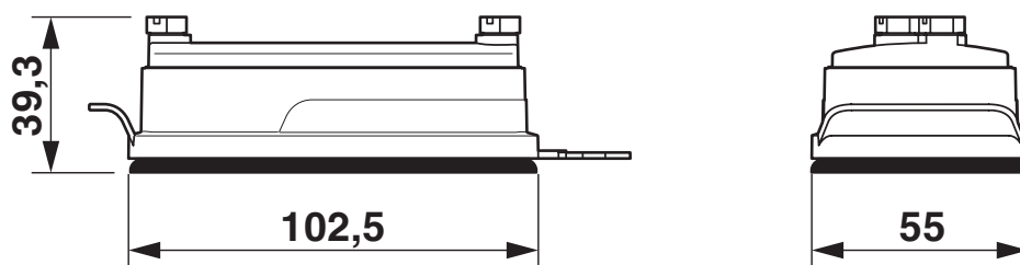
Rysunek wymiarowy
