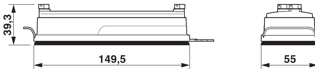
Rysunek wymiarowy
