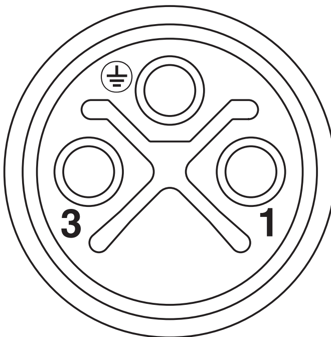
Rysunek schematyczny
