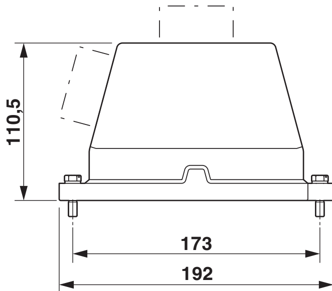
Rysunek wymiarowy
