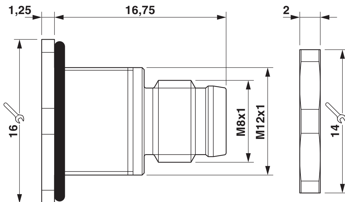
Rysunek wymiarowy
