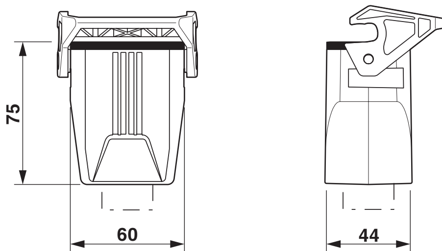
Rysunek wymiarowy
