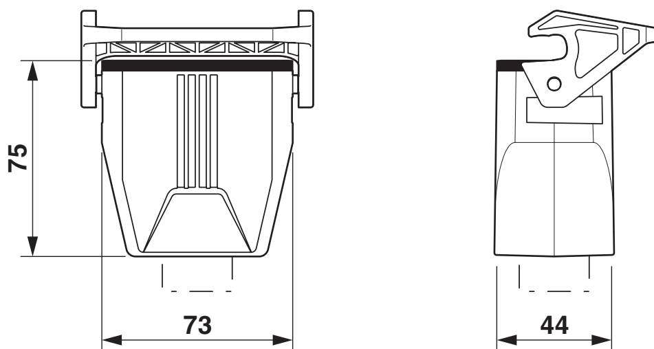
Rysunek wymiarowy
