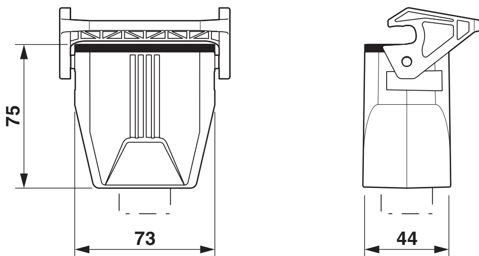
Rysunek wymiarowy
