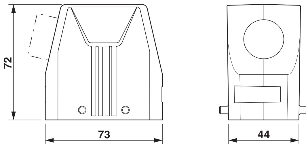
Rysunek wymiarowy
