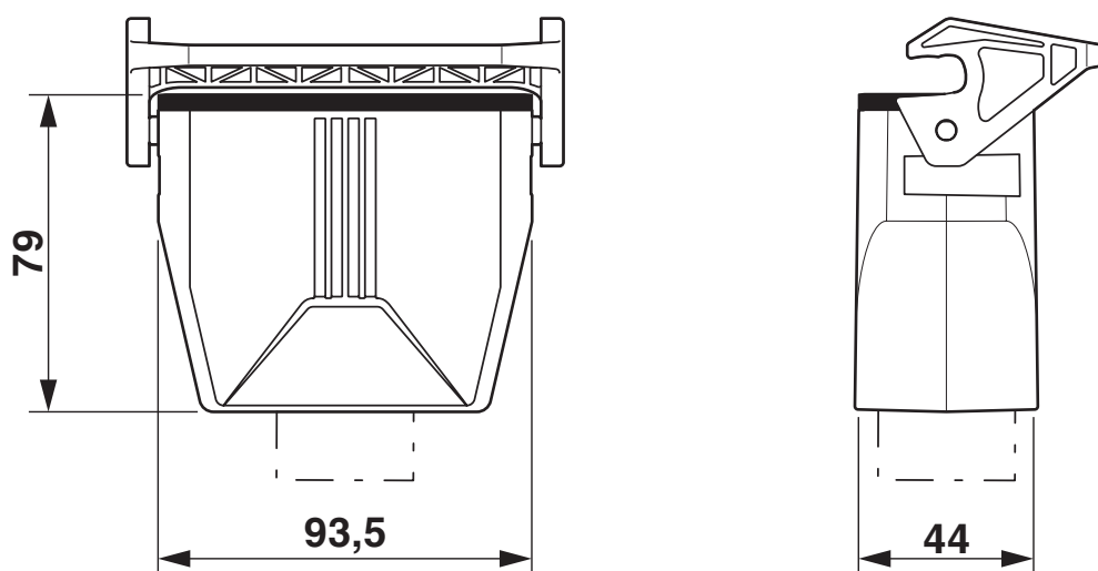
Rysunek wymiarowy
