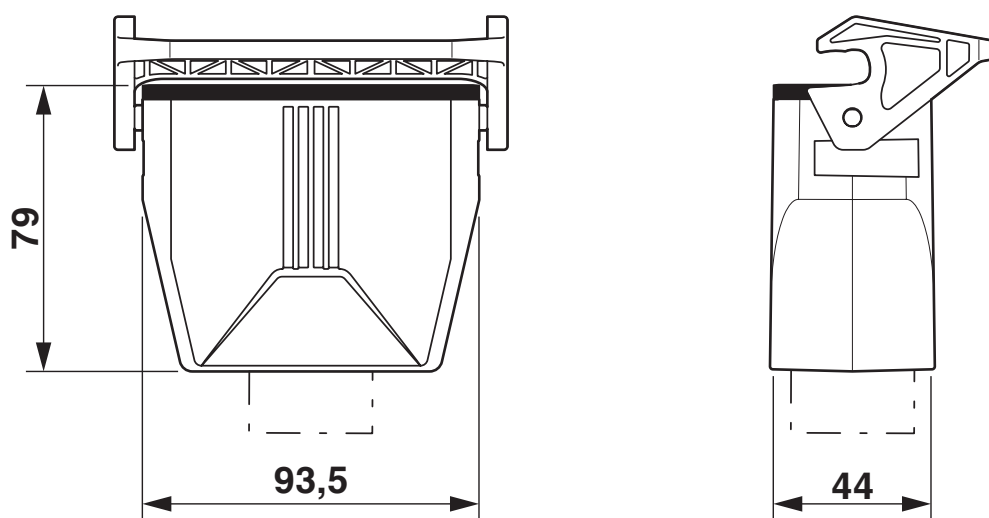
Rysunek wymiarowy
