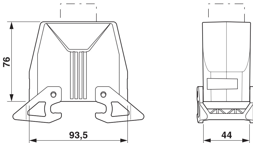
Rysunek wymiarowy
