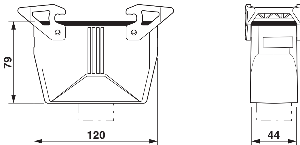
Rysunek wymiarowy
