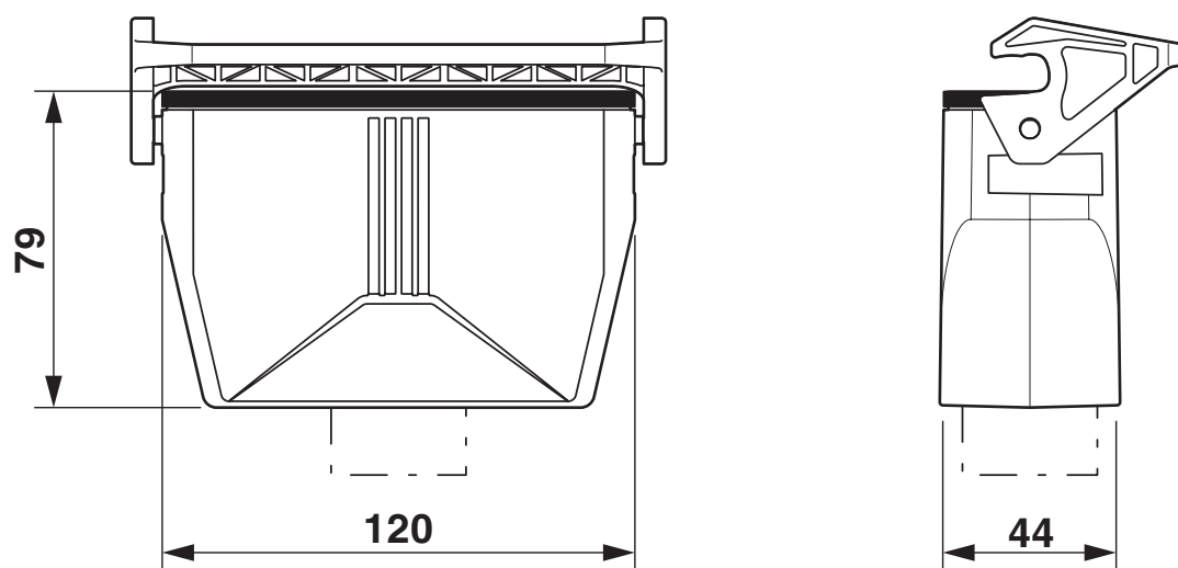
Rysunek wymiarowy
