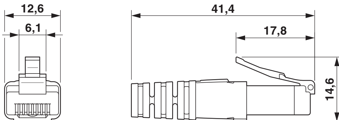
Rysunek wymiarowy
