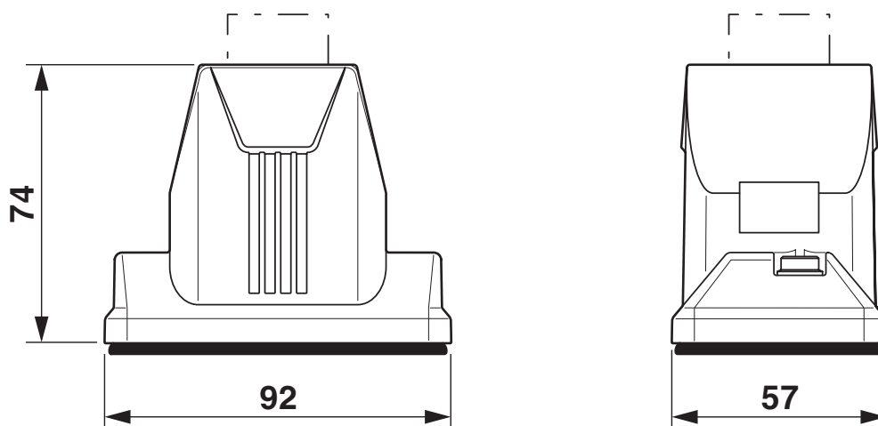
Rysunek wymiarowy
