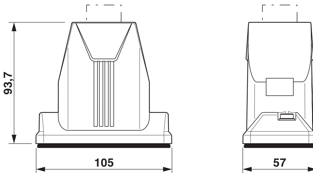
Rysunek wymiarowy
