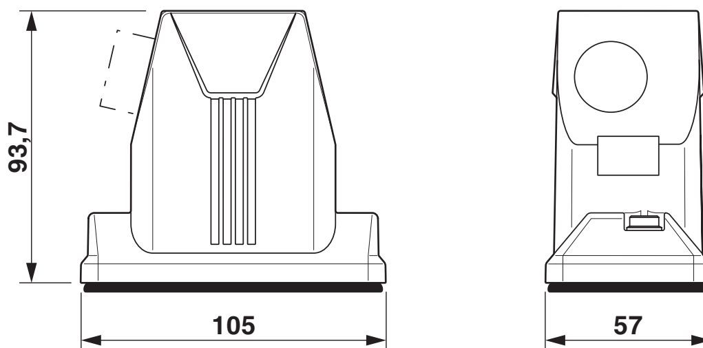
Rysunek wymiarowy
