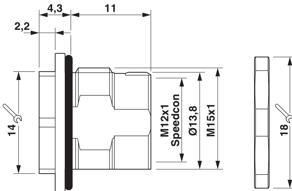
Rysunek wymiarowy
