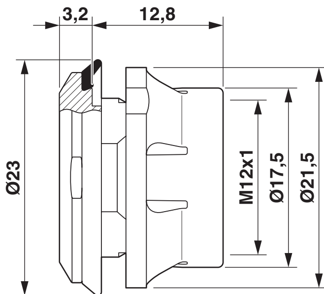
Rysunek wymiarowy
