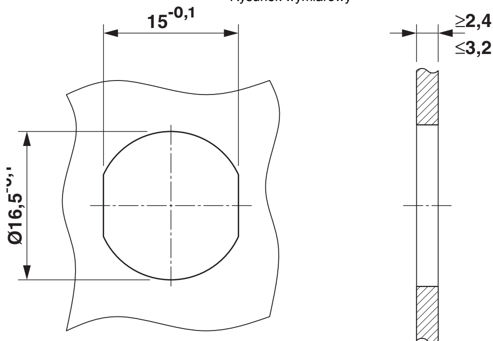
Otwór montażowy
