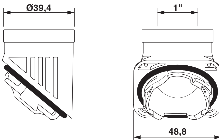
Rysunek wymiarowy
