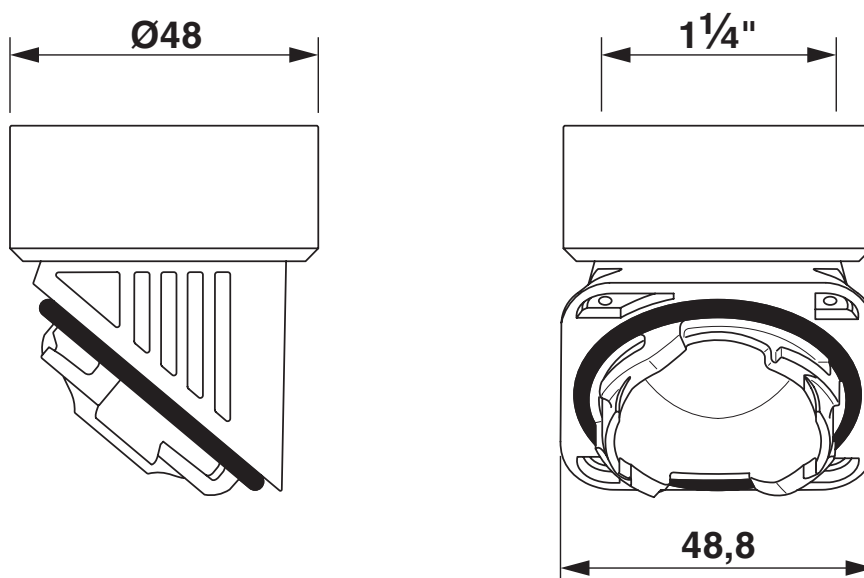
Rysunek wymiarowy
