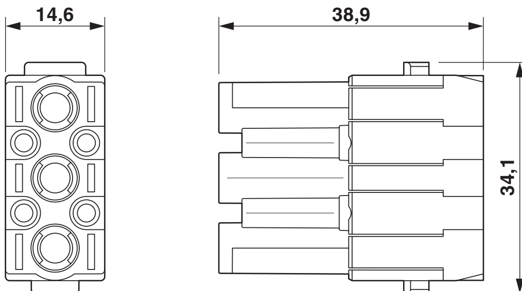
Rysunek wymiarowy
