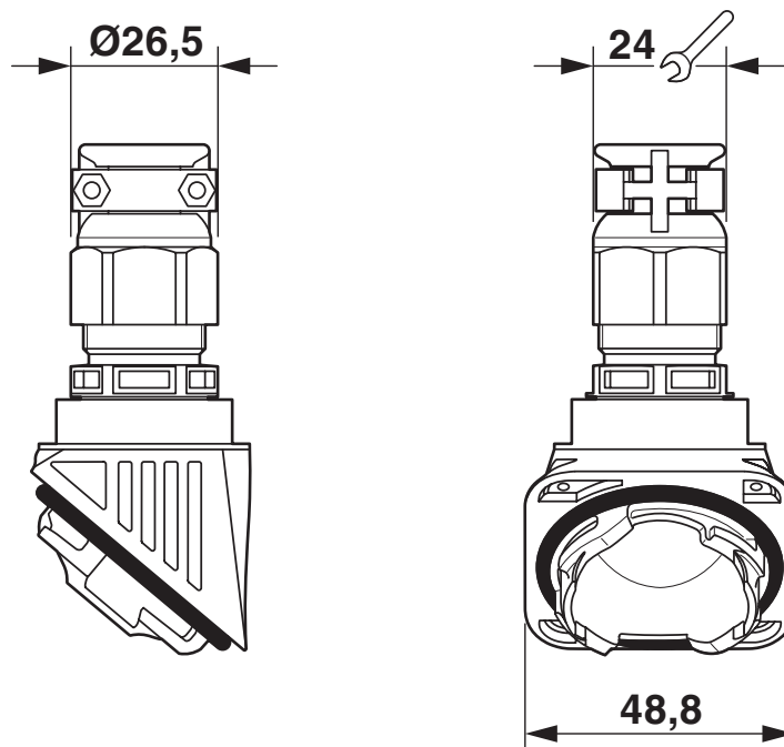
Rysunek wymiarowy
