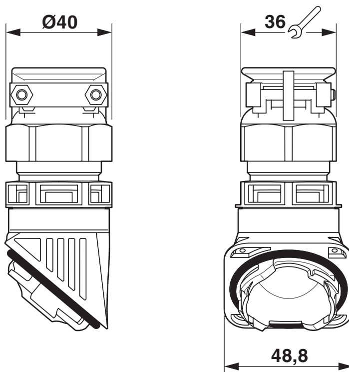
Rysunek wymiarowy
