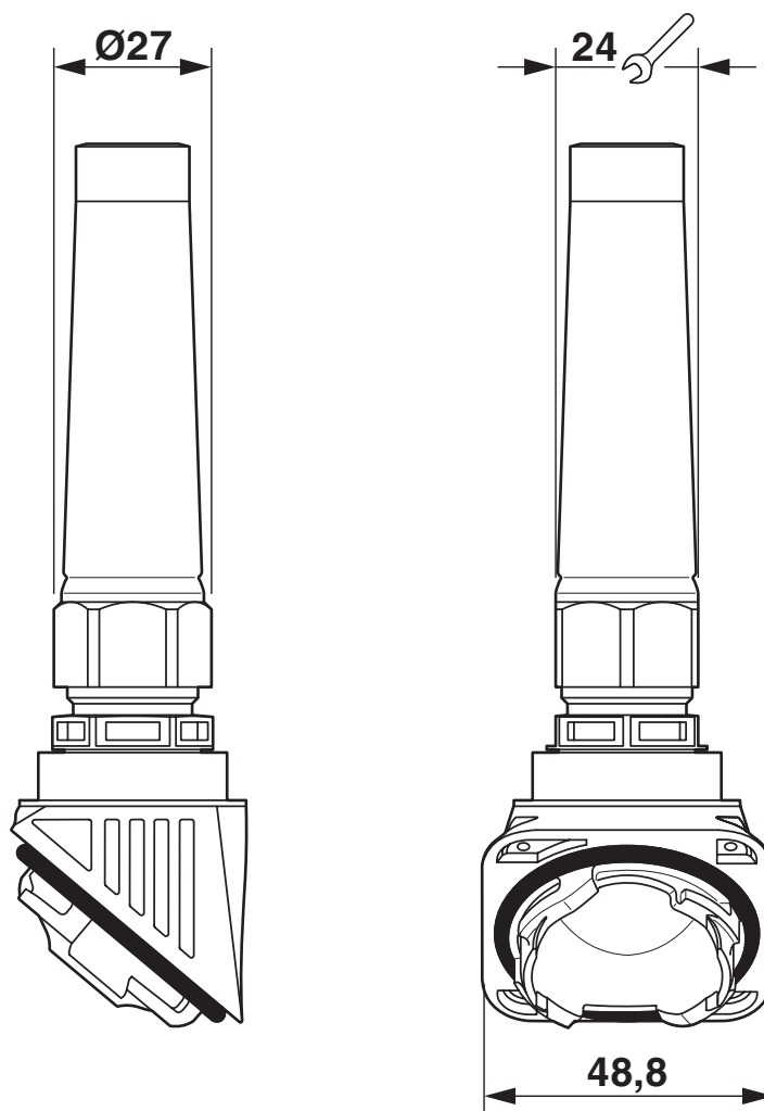
Rysunek wymiarowy
