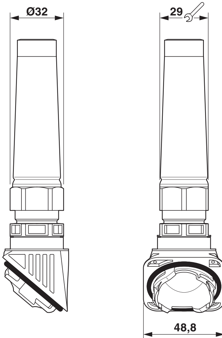
Rysunek wymiarowy
