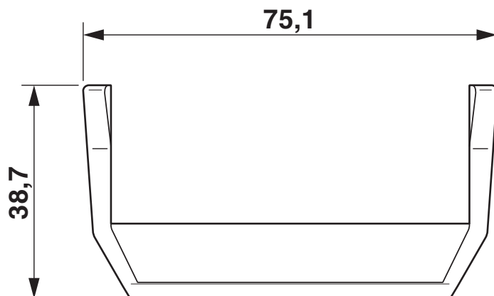
Rysunek wymiarowy
