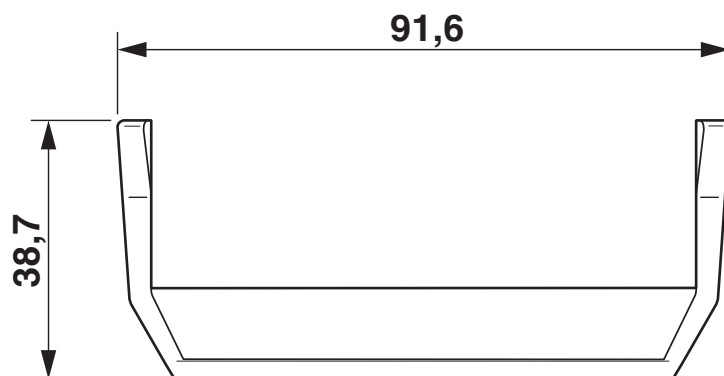
Rysunek wymiarowy
