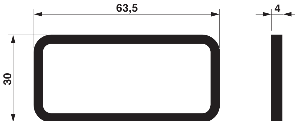
Rysunek wymiarowy
