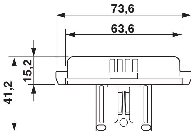
Rysunek wymiarowy
