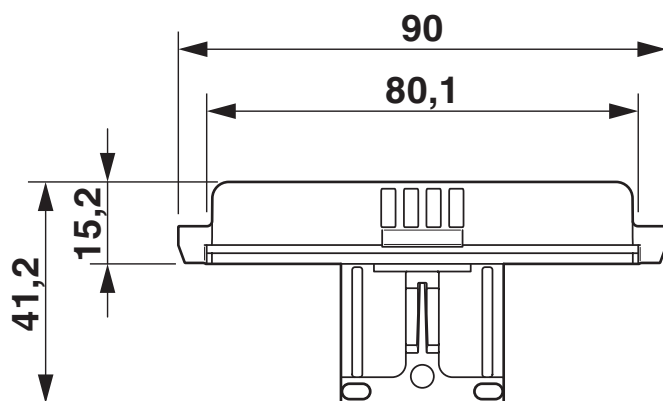
Rysunek wymiarowy
