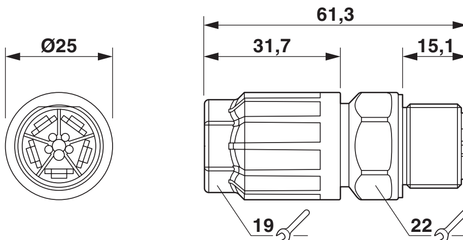
Rysunek wymiarowy
