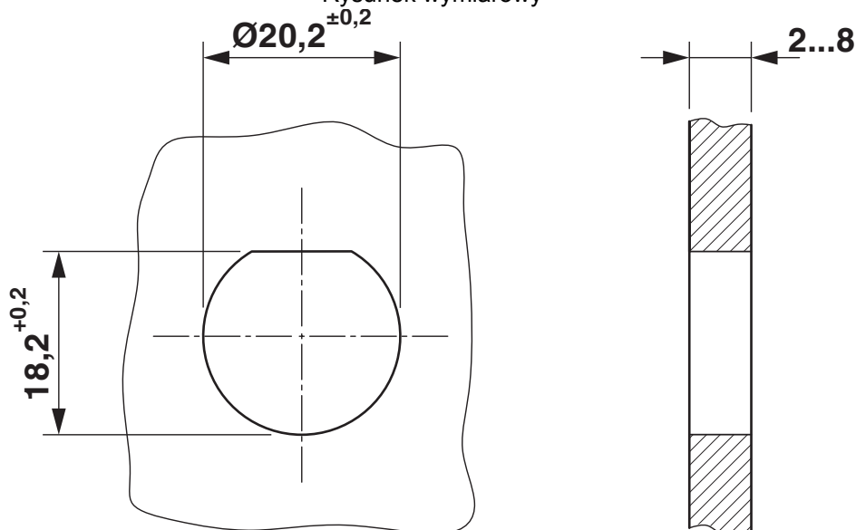
Rysunek wymiarowy
