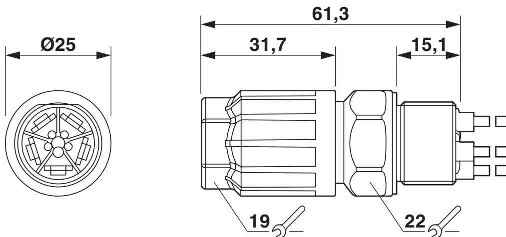
Rysunek wymiarowy
