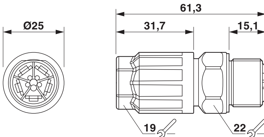
Rysunek wymiarowy
